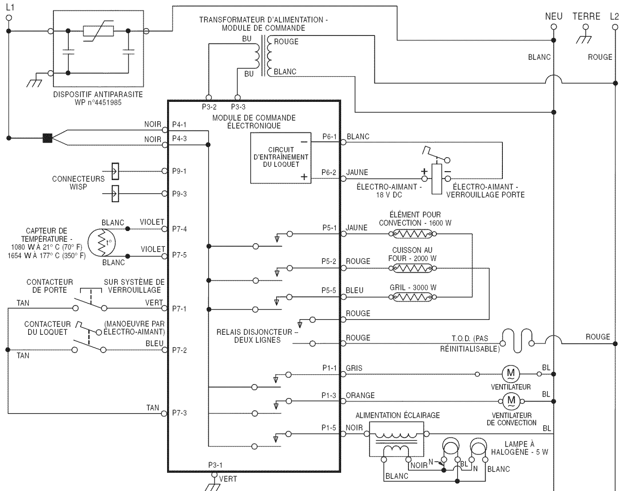
Schéma du four (Oven wiring diagram).
