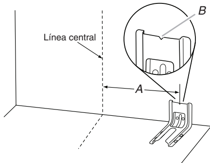
A. 12^{53/64} " (32,6 cm) B. Muesca en V del soporte
