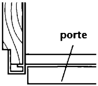
panneau latéral hors de la pièce de garniture latérale, et en retrait.
