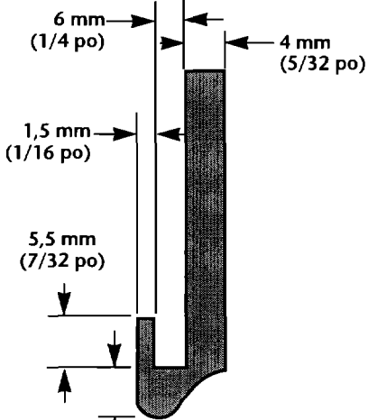
Vue de l'extrémité de la pièce de garniture latérale
