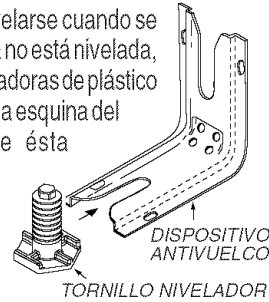
TORNILLO NIVELADOR
