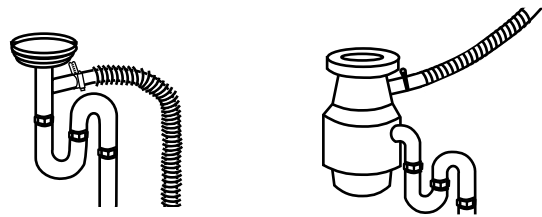
Conexión de desagüe - a la T de desagüe
