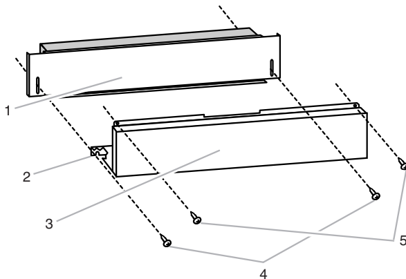
1. Panel inferior 2. Sujetador de puesta a tierra 3. Panel de acceso 4. 2 tornillos inferiores 5. 2 tornillos superiores
