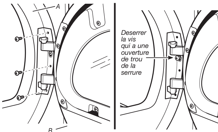
A. Panneau avant du sèche-linge B. Armature de la porte
