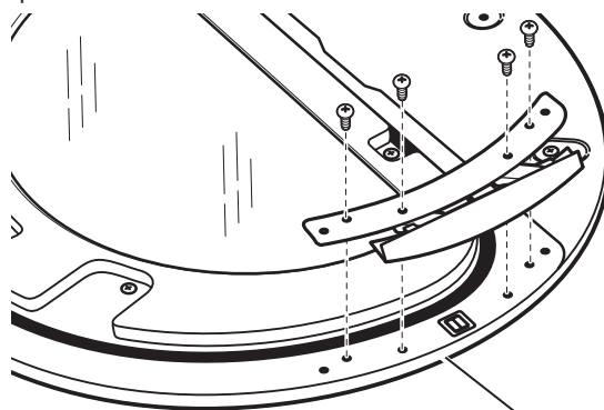
Cerniere sportello
