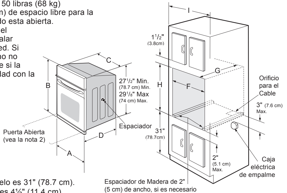
Figura 1 HORNO SENCILLOS DE PARED DE 24"
