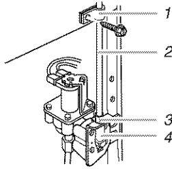
1. Bride du tube 2. Tube en plastique 3. Écrou de compression 4. Entrée d'eau de la valve
