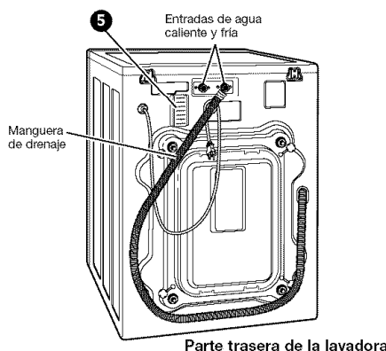
Parte trasera de la lavadora
