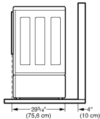
Dimensiones requeridas para la instalación con pedestal
