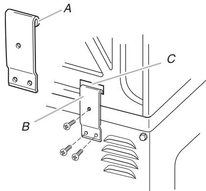
A. Extremo en forma de gancho B. Soporte para apilar C. Ranura en la parte posterior de la secadora
