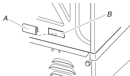
A. Garniture de plastique B. Fente
