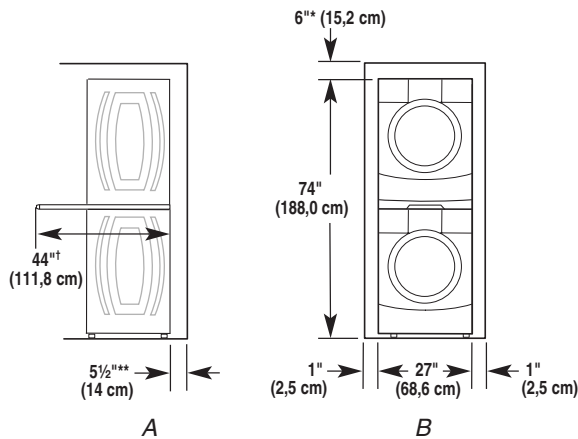
A. Vue latérale - laveuse et sècheuse superposées B. Vue de face - laveuse et sècheuse superposées
