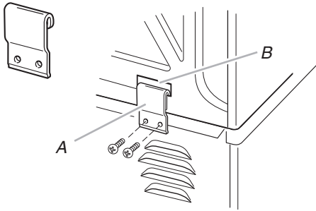
A. Bracket B. Slot
