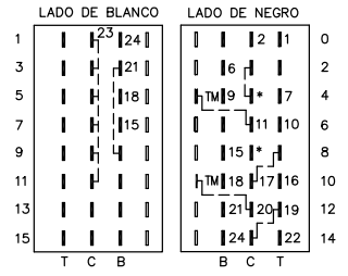
DIAGRAMA DE CONEXIONES NO. DE PIÉZA 137394100 A
